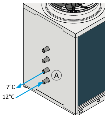
Verbraucher- Kühlung
