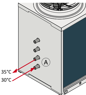
Verbraucher- Heizung
